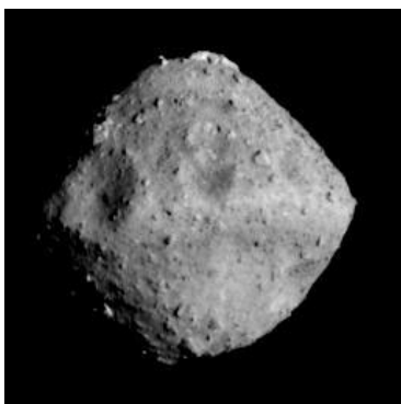
小惑リュウグウ（提供：JAXA、東大など）
